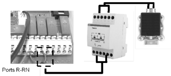
Figure 41. Branchement de l'électrovanne
