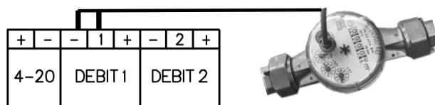
Figure 39. Branchement du compteur d'eau sur entrée débit 1 (fil rouge sur borne 1 et fil noir sur borne -)
