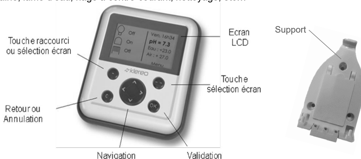
Figure 6. Ecran et touches de navigations de la commande déportée Klereo PAD
