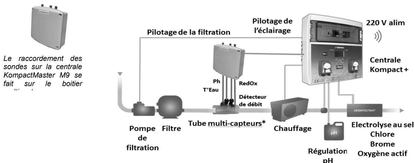
Figure 10. Diagramme d'installation Compact Master
