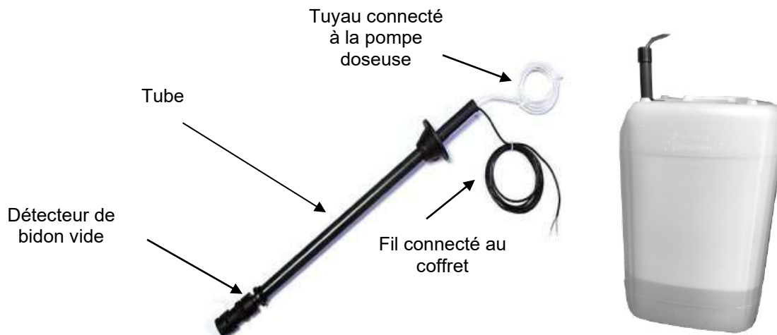
Figure 24. détecteur bidon vide
