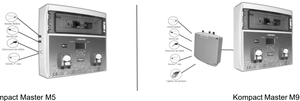
Figure 30. Branchement des capteurs sur la centrale Kompact Master
