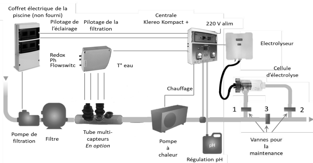
Figure 29. Installation de la cellule d'électrolyseur
