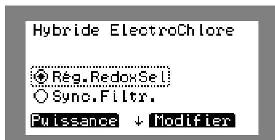
Figure 58. Réglage de la puissance de fonctionnement de l'électrolyseur
