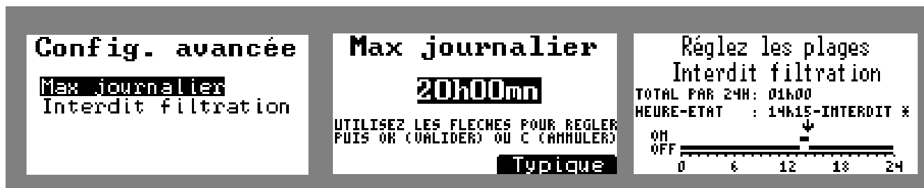
Figure 51. Configuration avancée de la filtration en mode régulé : max jour et interdit filtration
