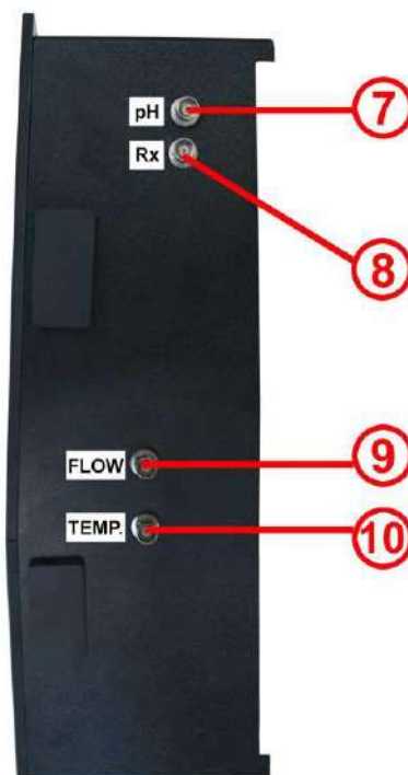
Figure : boîtier du régulateur vu du côté droit
