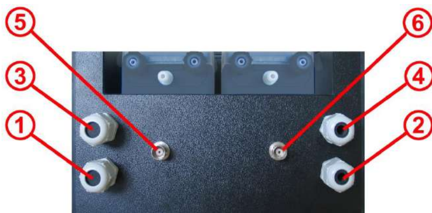
Figure : boîtier du régulateur vu d'en bas
