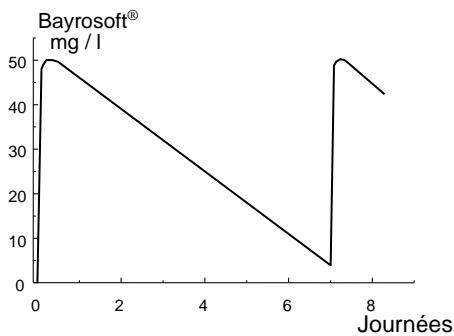
Dosage automatique à 24 °C (Evolution de la concentration de Bayrosoft® au cours d'une semaine)
